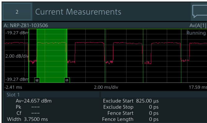
Измерение таймслотов сигнала Bluetooth® с исключением начального времени
